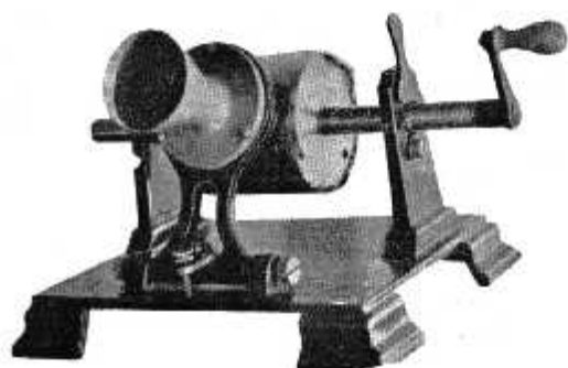
DE EERSTE EDISON „GRAMOFOON“
